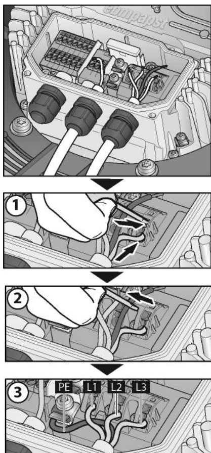
Kuva 2: Johtojen kiinnitys liittimiin
