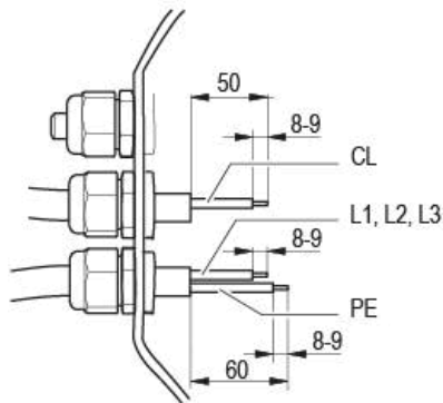
Kuva 1: Suositut kuorimismitat mm:inä (kytkentärasia) seloste: CL=säätöjohtimet
