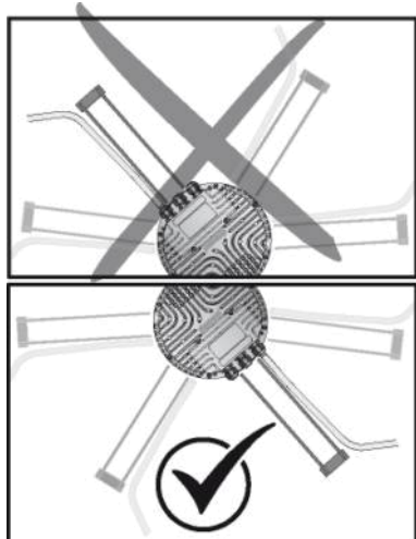
Kuva 3: Kaapelien asennus pystyasentoon asennettuihin puhaltimiin.
