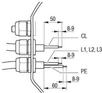
Kuva 1: Suositellut kuorimismitat mm:inä (kytkentärasia) seloste: CL=säätöjohtimet
