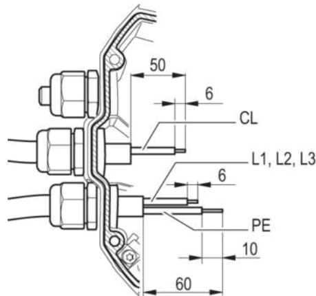
Kuva 1: Suositut kuorimispituudet mm:inä (kytkentärasiasa) seloste: CL=säätöjohtimet
