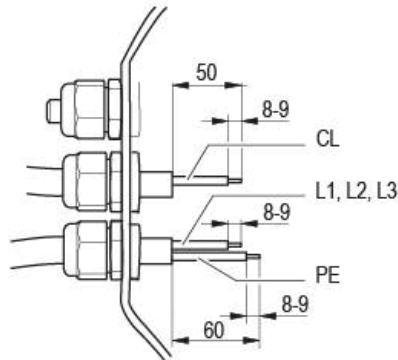
Kuva 1: Suositut kuorimispituudet mm:einä (kytkentärasiasa) seloste: CL=säätöjohtimet
